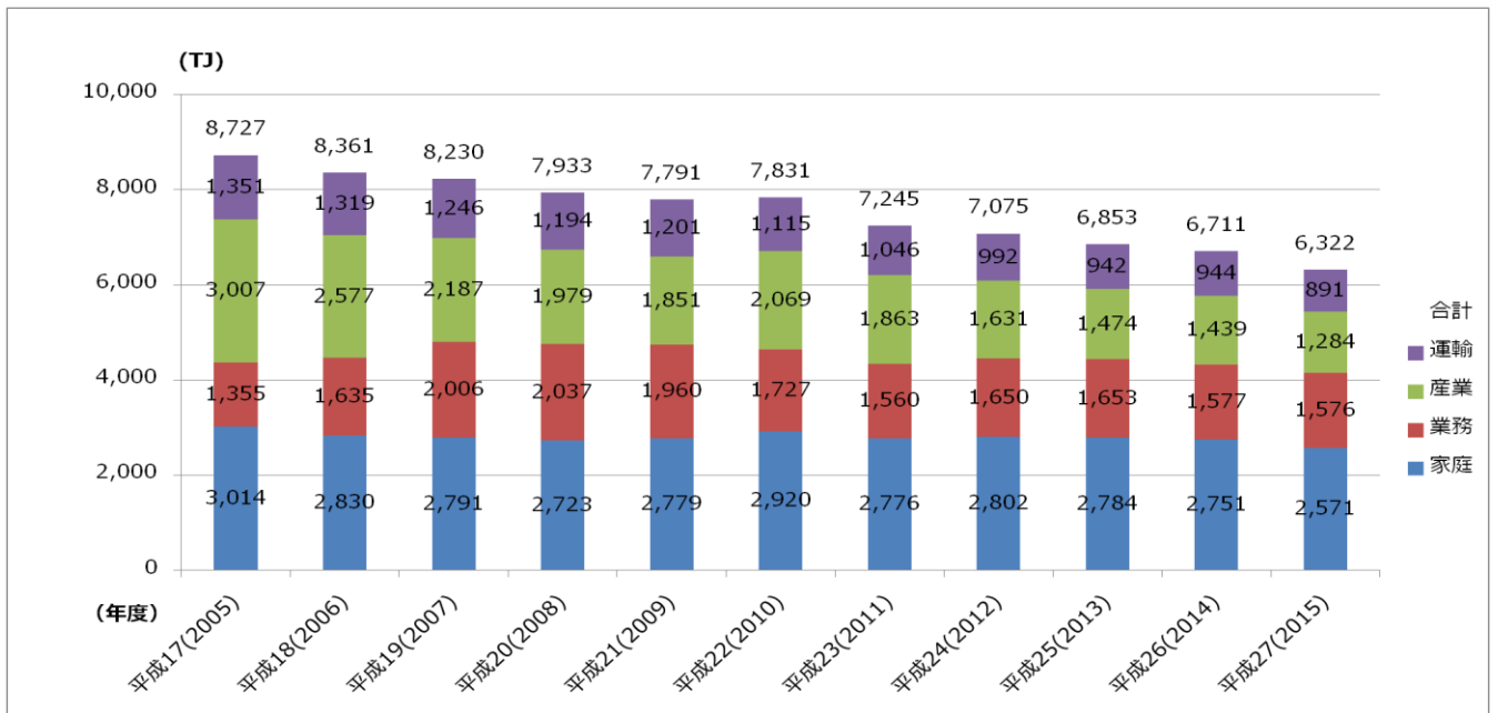
図 2 小平市の部門別エネルギー消費量の推移
